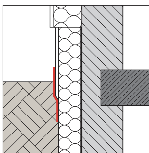
Stucafdichting
